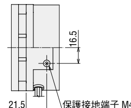
保護接地端子詳圖
