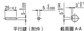
平行鍵 (附件)
