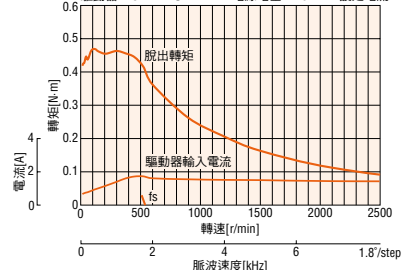
PKP245D23A2/ PKP245D23B2
