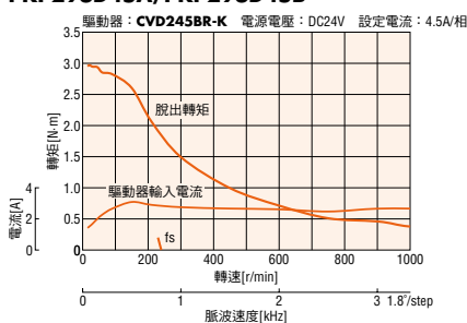
PKP296D63A/PKP296D63B
