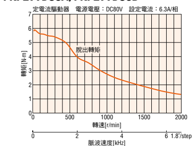
PKP299D63A/PKP299D63B
